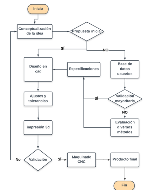
Fig. 6 Diagrama de flujo del caso de aplicación, losetas. Elaboración propia
