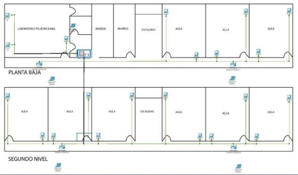
Fig. 3. Mapeo de nodos de red del nuevo edificio.
