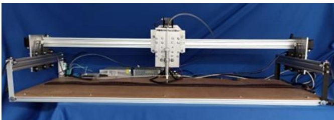
Figura 15: Prototipo diseñado.
